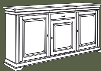
Art. 0790 Credenzona 3 porte liscio L. 228 P. 52 H. 112 Peso kg 100,00 - mc 1,46
