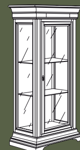
Art. 0768 Vetrinetta a 1 porta con piano a bacheca liscia L. 64 P. 42 H. 140 Peso kg 20,00 - mc 0,42
