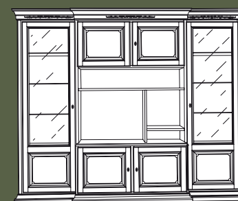
Art. 0732/B Composizione intagliata L. 295 P. 58 H. 242 Peso kg 170,00 - mc 2,31
