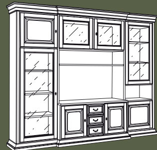
Art. 0782/A Composizione liscia L. 295 P. 58 H. 242 Peso kg 170,00 - mc 2,31
