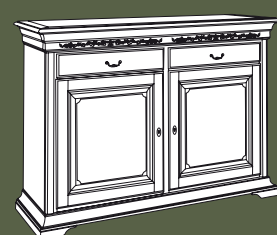
Art. 0741 Credenzona 2 porte intagliato L. 158 P. 52 H. 112 Pag. 19 Peso kg 65,00 - mc 1
