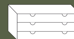
Art. 0725/C1 Cassettiera interna 3 cassetti L. 106 P. 46 H. 45 Pag. 58 Peso kg 15,00 - mc 0,25
