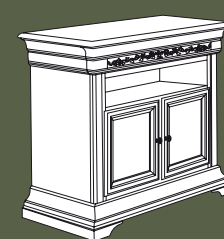
Art. 0716 Porta TV intagliato L. 87 P. 45 H. 77 Pag. 20 Peso kg 25,00 - mc 0,33
